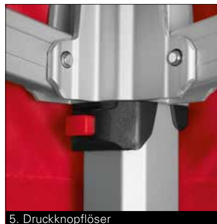
5. Druckknopflöser
